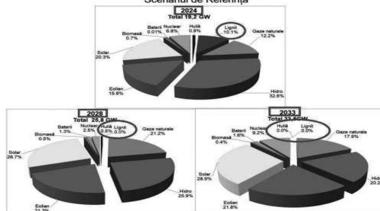
Fig.5.3.5 Structura capacității de producere nete disponibile în SEN Scenariul de Referință
